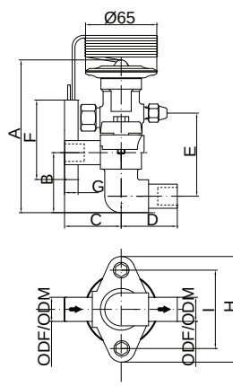
TRFE直通型热力膨胀阀
